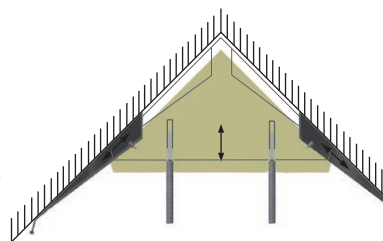
Schnittansicht 2:
