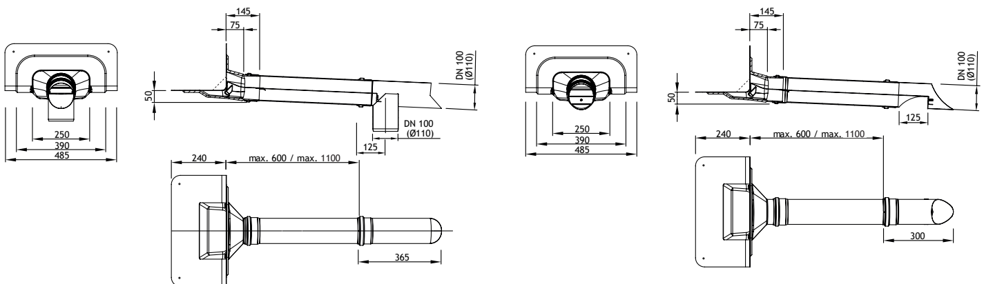
Attika-Meso-2-Gully mit Keil, mit Stromteilabzweig (kurze Version) Art.Nr.: 3215.BIT
