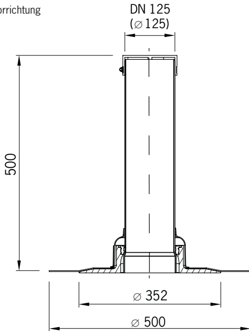
Durchgriffvorrichtung Ø DN 125
